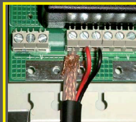
Klemmen für Video+DC
